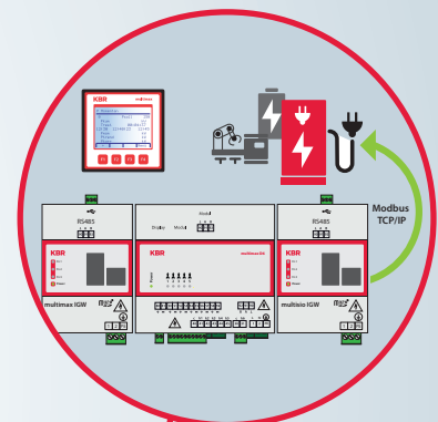
multimes IGW intelligentes Gateway speziell für die Anbindung von zu regelnden Lasten in Energieoptimierungsanlagen. Die perfekte Wahl für die Energieoptimierungs-Integration von Ladesäulen, Batteriespeichern und anderen steuerbaren Komponenten.
