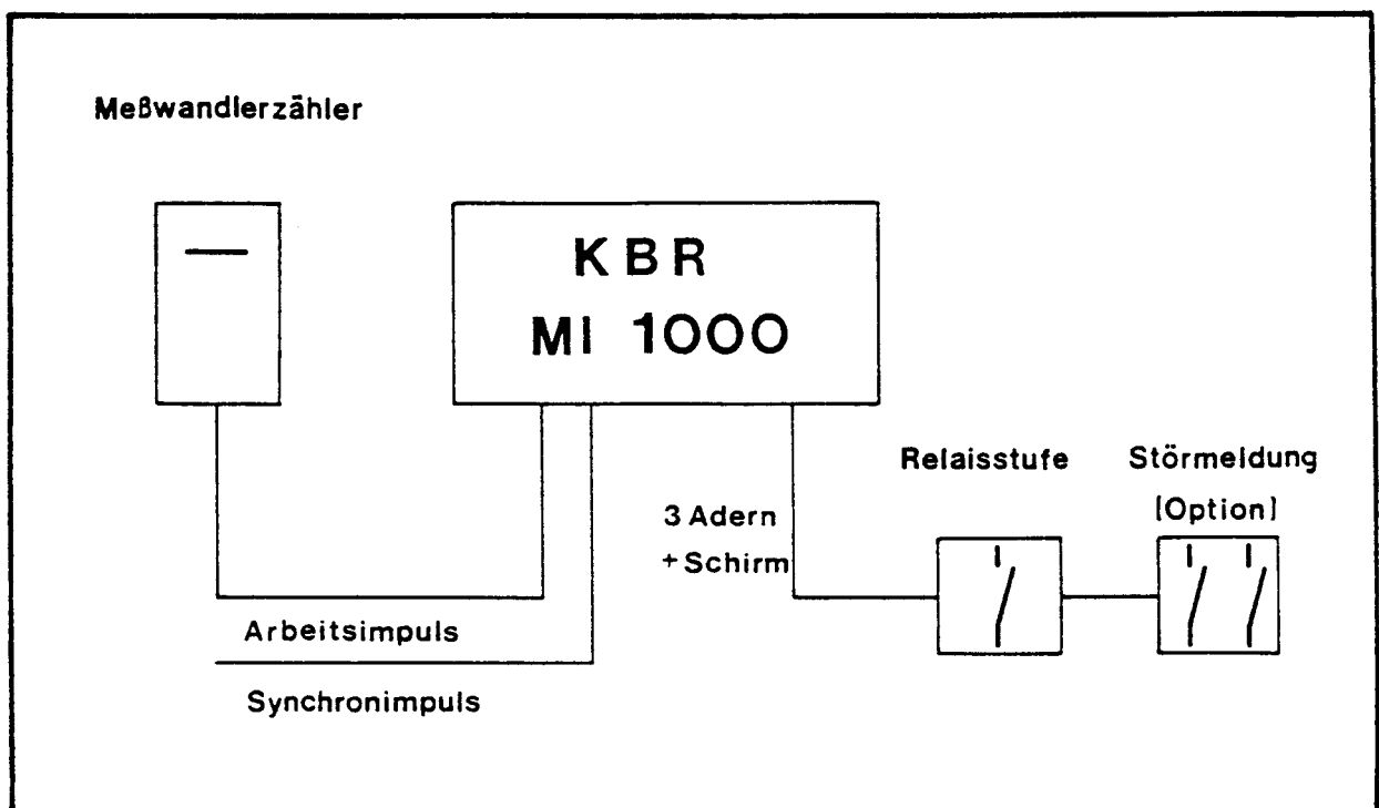
PRINZIPSCHALTBILD
