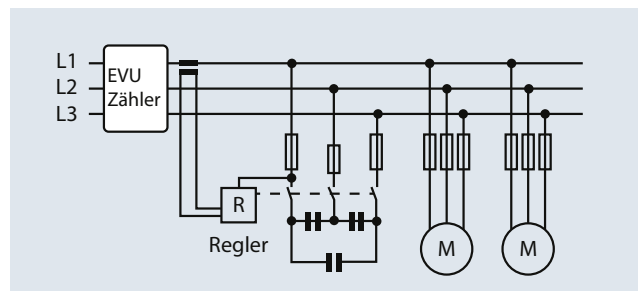
Bild 8: Schematischer Einbau einer Blindleistungskompensationsanlage
